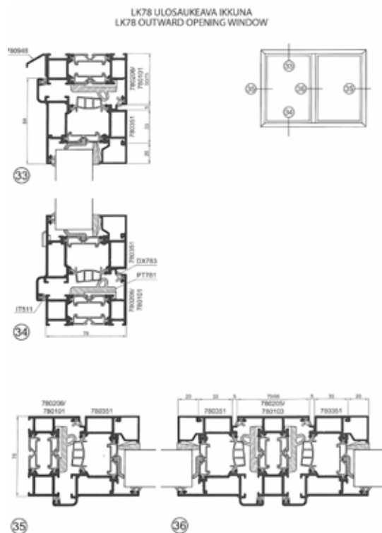
► Esimerkkikuva ikkunaprofiilista.
